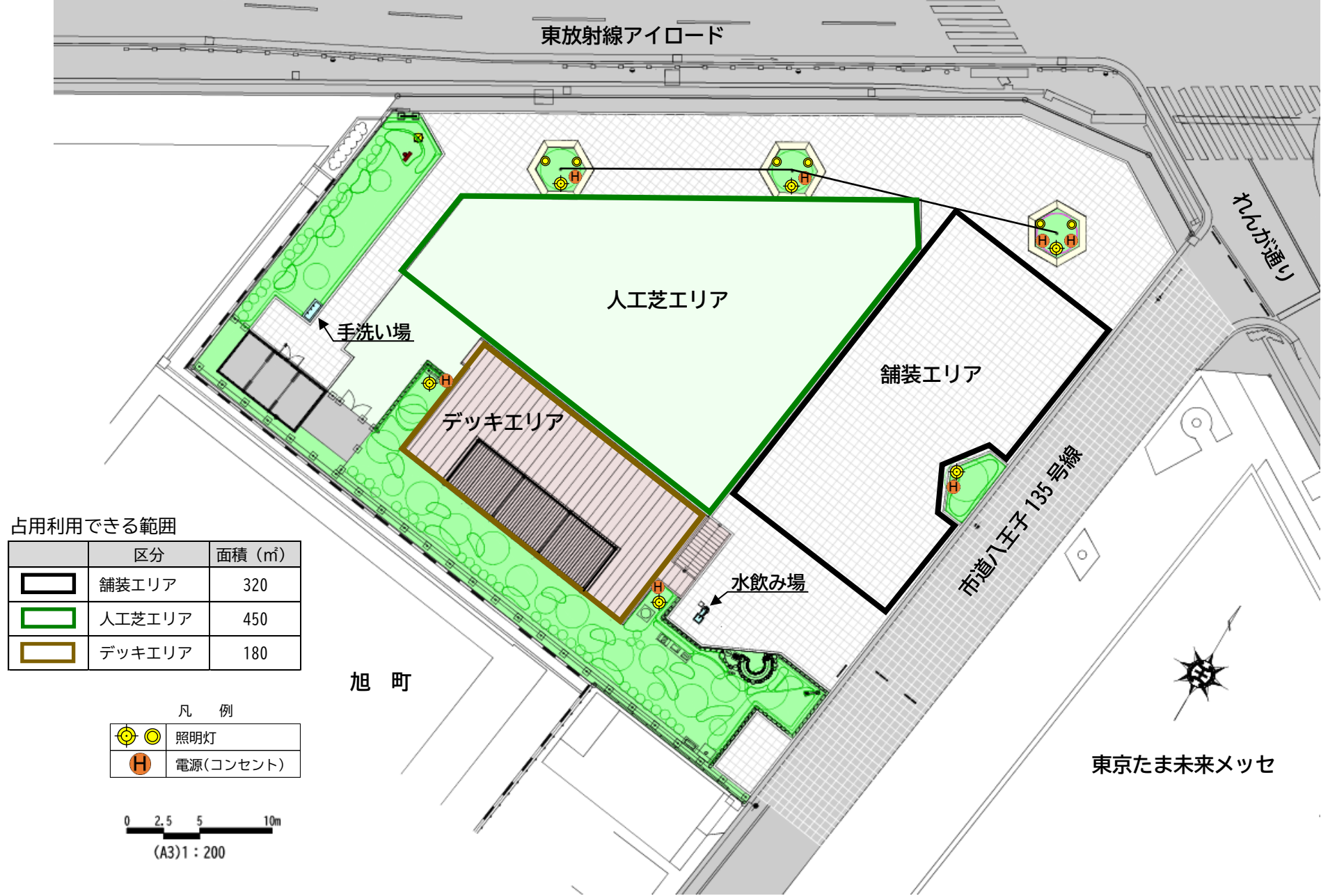
別図（平面図）
